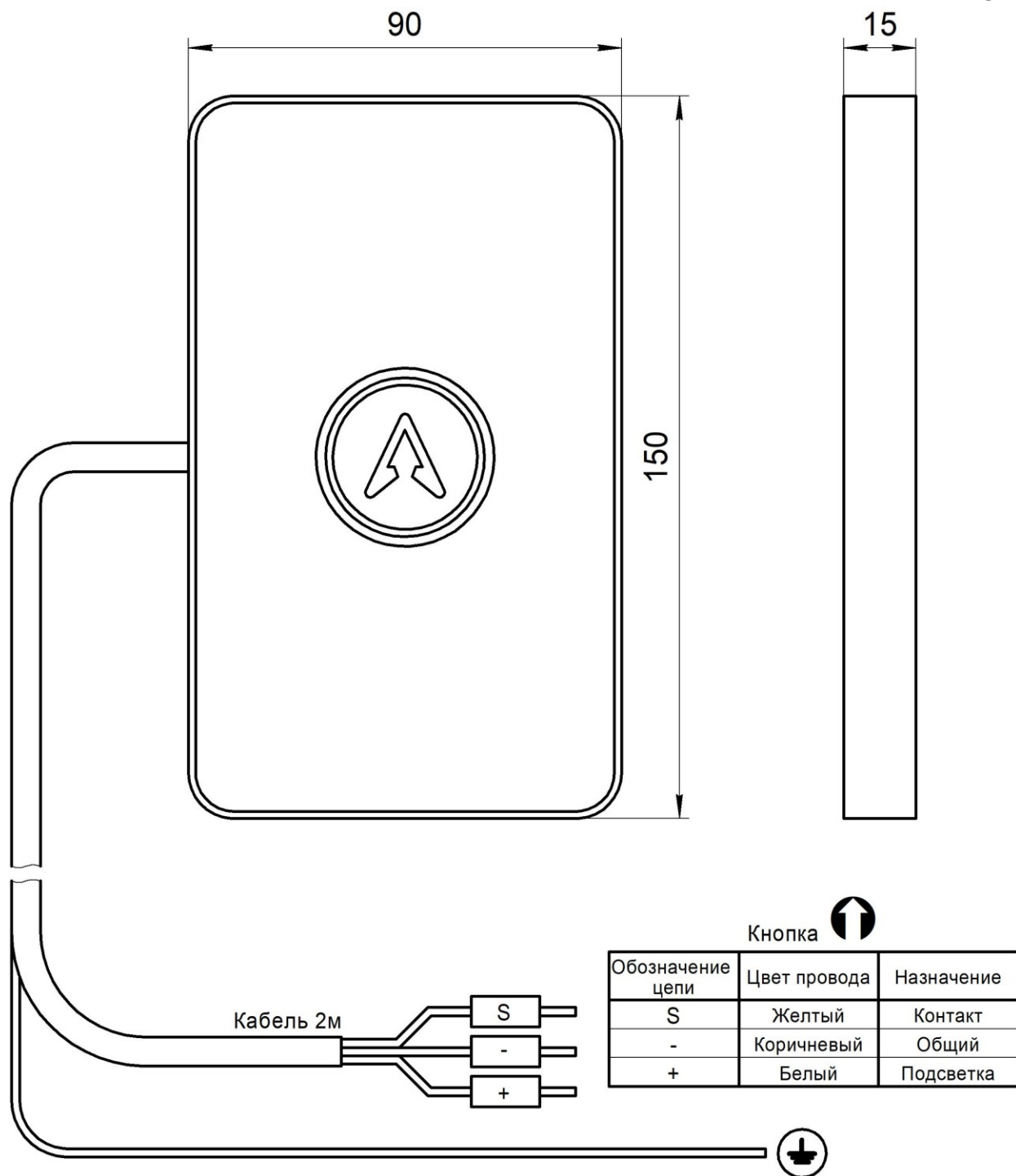
Рис.1 Внешний вид и габаритные размеры Вызывного поста ОНИКС НШЕК.468381.123-01
